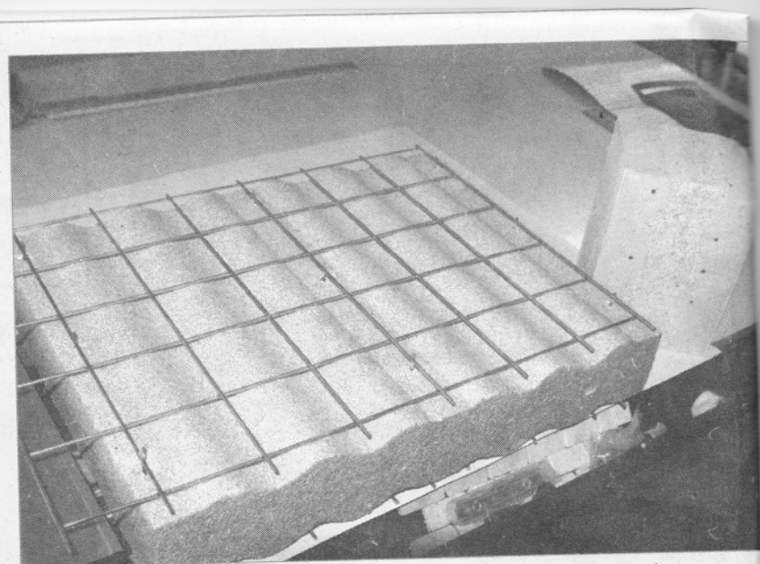
Τα ειδικά πάνελ και τούβλα που χρησιμοποιούνται για τη μόνωση
